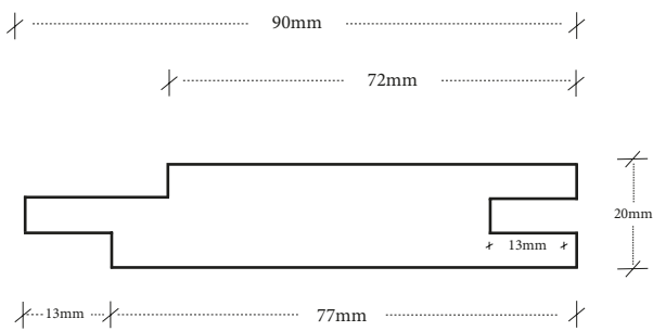
GT 12 20x90 (77mm)
